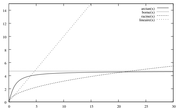
FIGURE A.4: Fonctions de répartition concave bornée (arc tangent) et non bornée (racine carrée)
