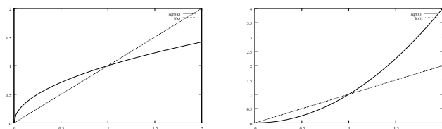
FIGURE 1.1: Fonctions de répartition concave (à gauche) et convexe (à droite)
